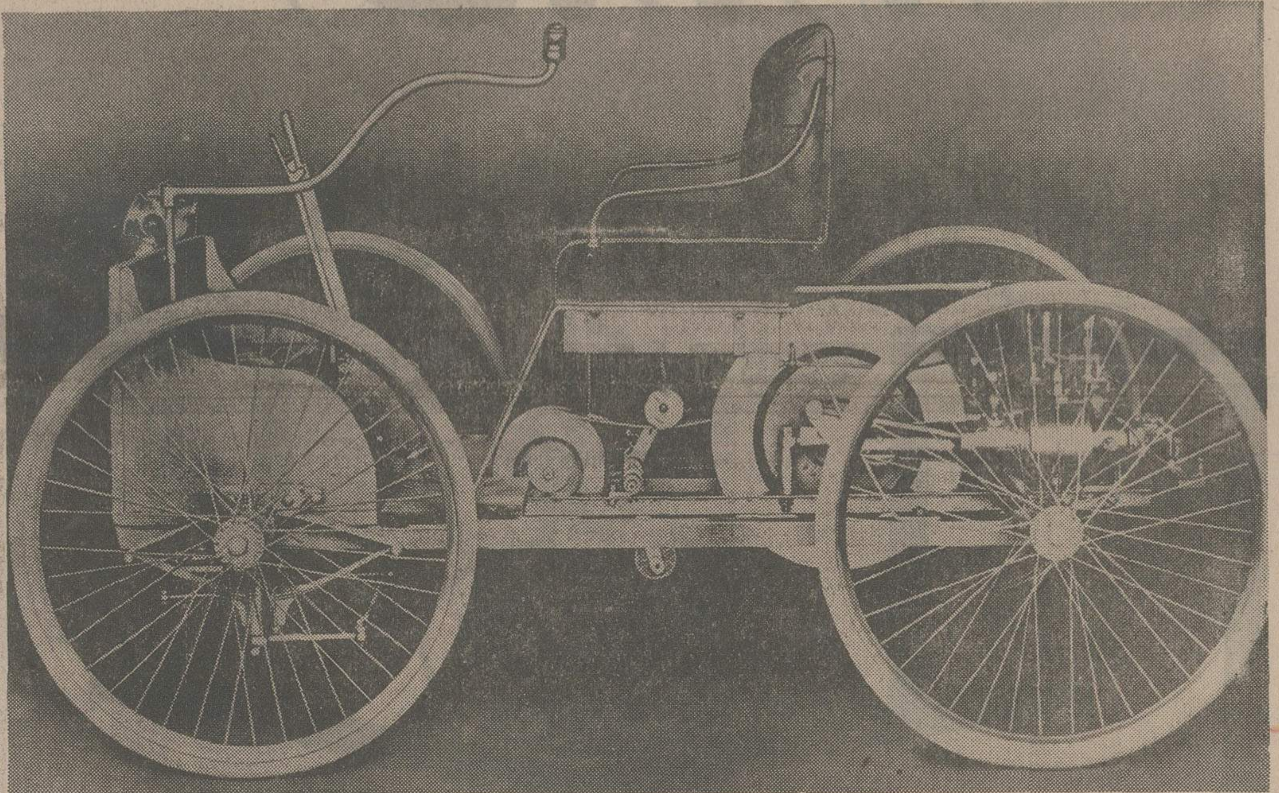
اولین اتومبیلی که «هنری فورد» در سال ۱۸۹۶ ساخت که موتور آن ۲ سیلندر داشت و «فورد» شخصا آنرا با سرعت ۱۰ میل در ساعت حرکت درآورد.
