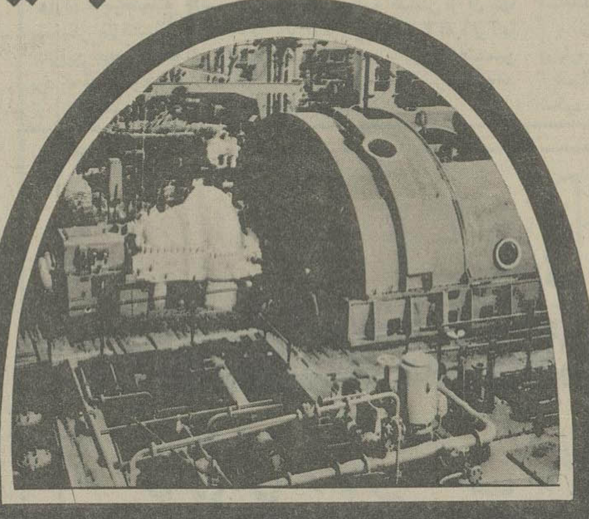
توربین بخار ۲۳۶ مگاواتی (هسته ای) برای طرح نیروگاه اتمی مدرس
