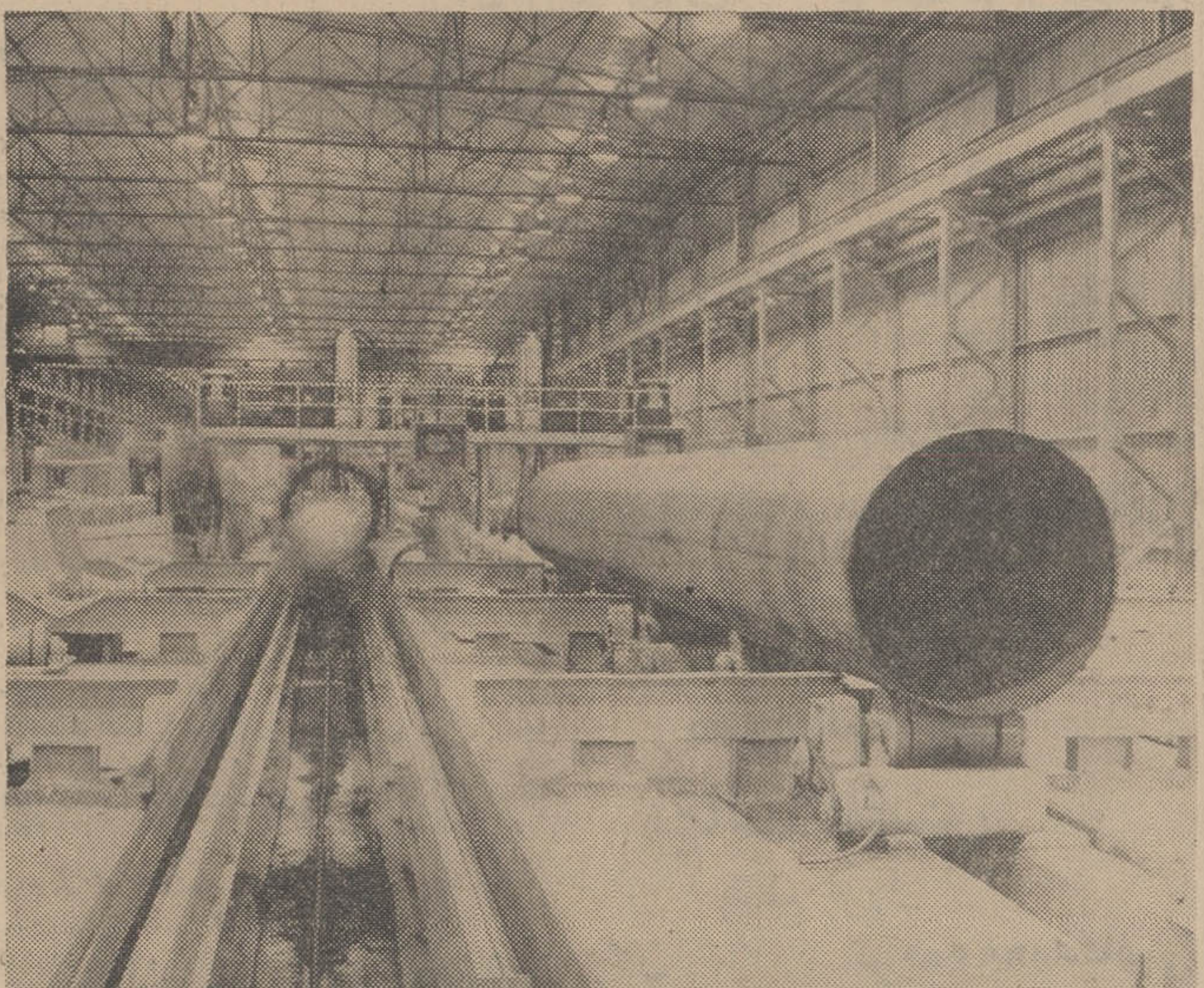
کارخانجات لوله سازی اهواز
