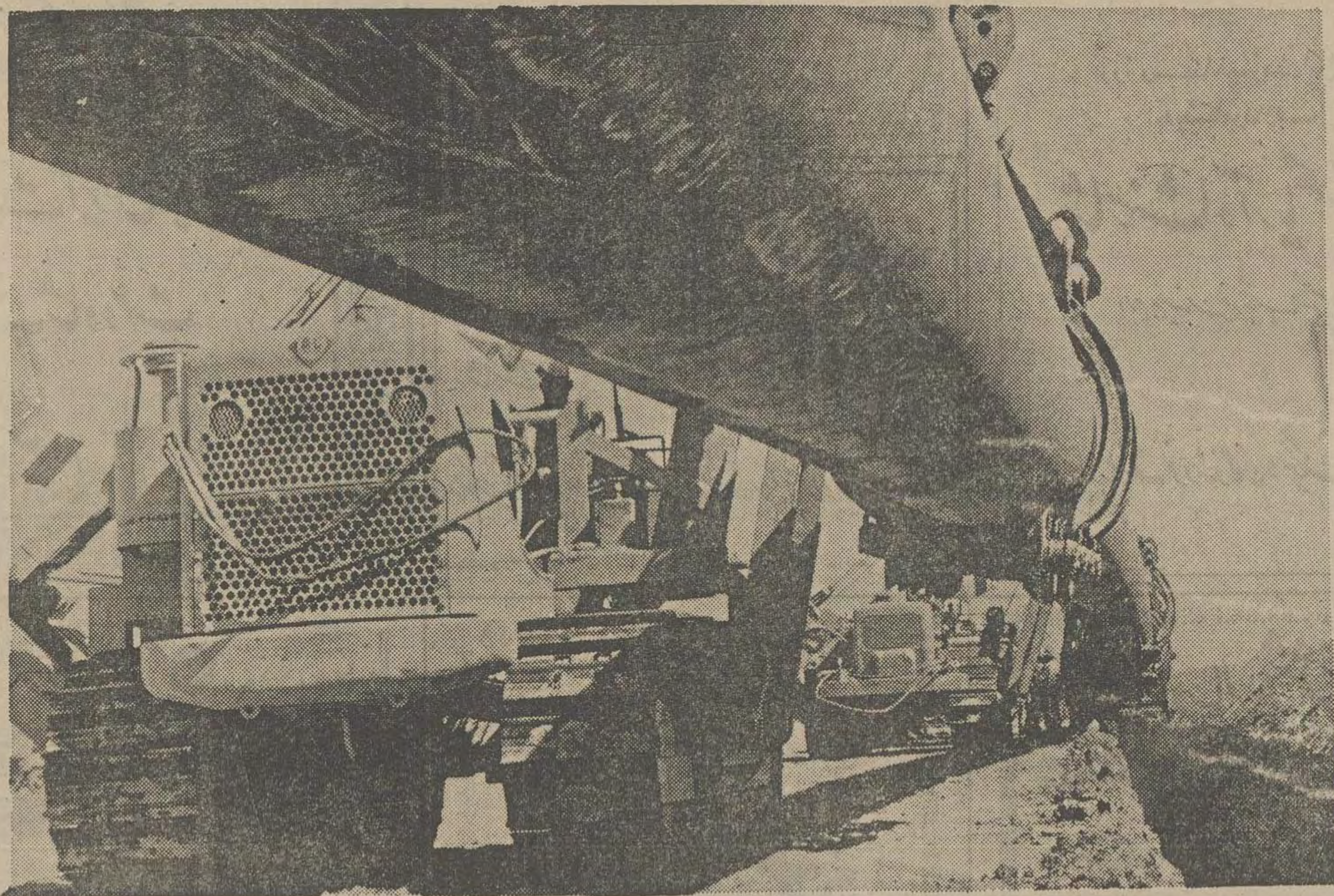
عملیات لوله‌گذاری شاه لوله گاز ایران
