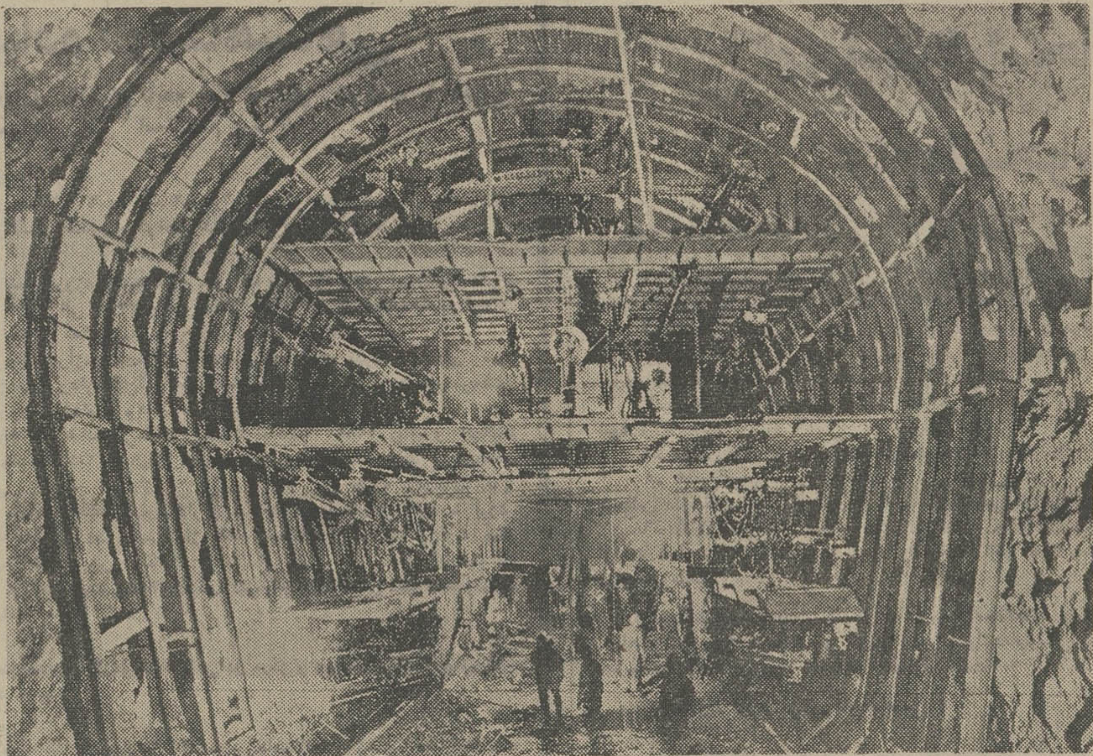
تونل شماره ۱۴ راه هر از که بهنگام ساختمان یش از ده نوبت ریزش کردو سرانجام با یکبار بردن روشی که عکس نشان می دهد، تونل مهار شدو ساختمان پویان رسید.
