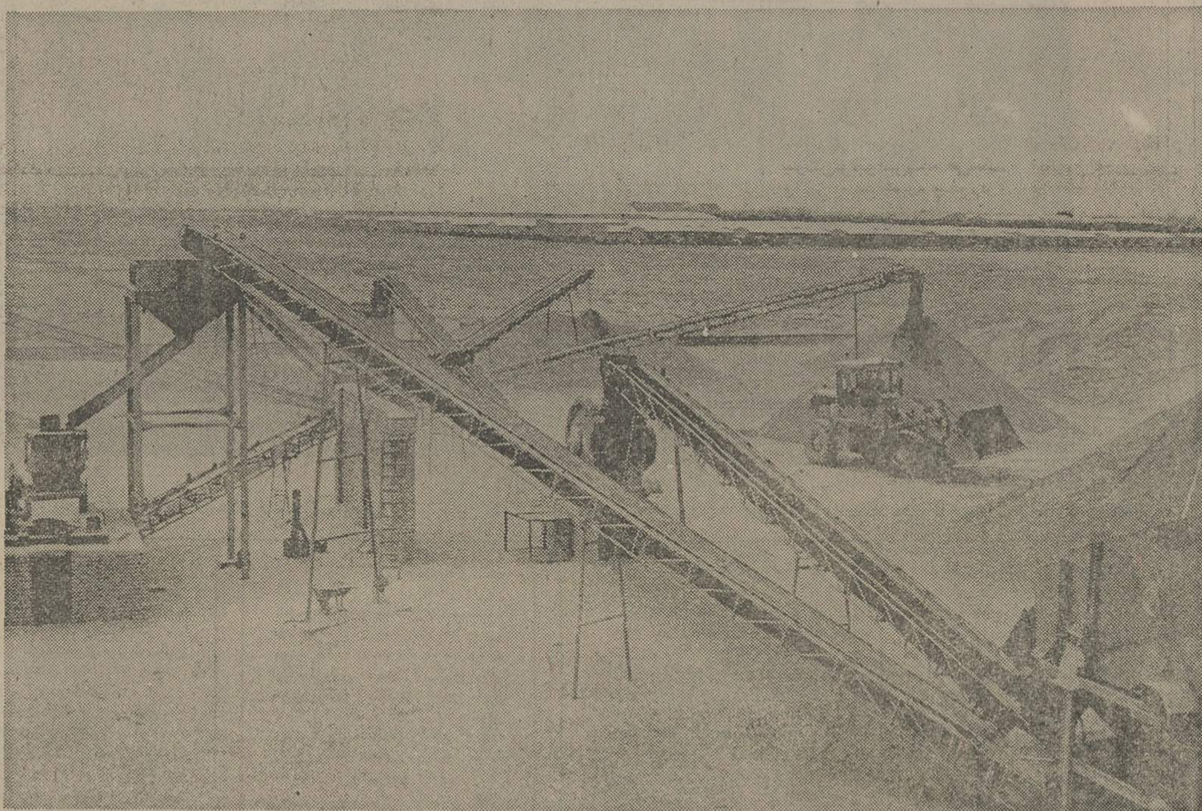
عملیات دانه بندی مصالح از سوی کنسرسیوم چهار راه با مدرنترین ماشین آلات صورت میگیرد تا هیچگونه تنطه ضعیفی از لحاظ زیرسازی ساختمان راهها نداشته باشد.
