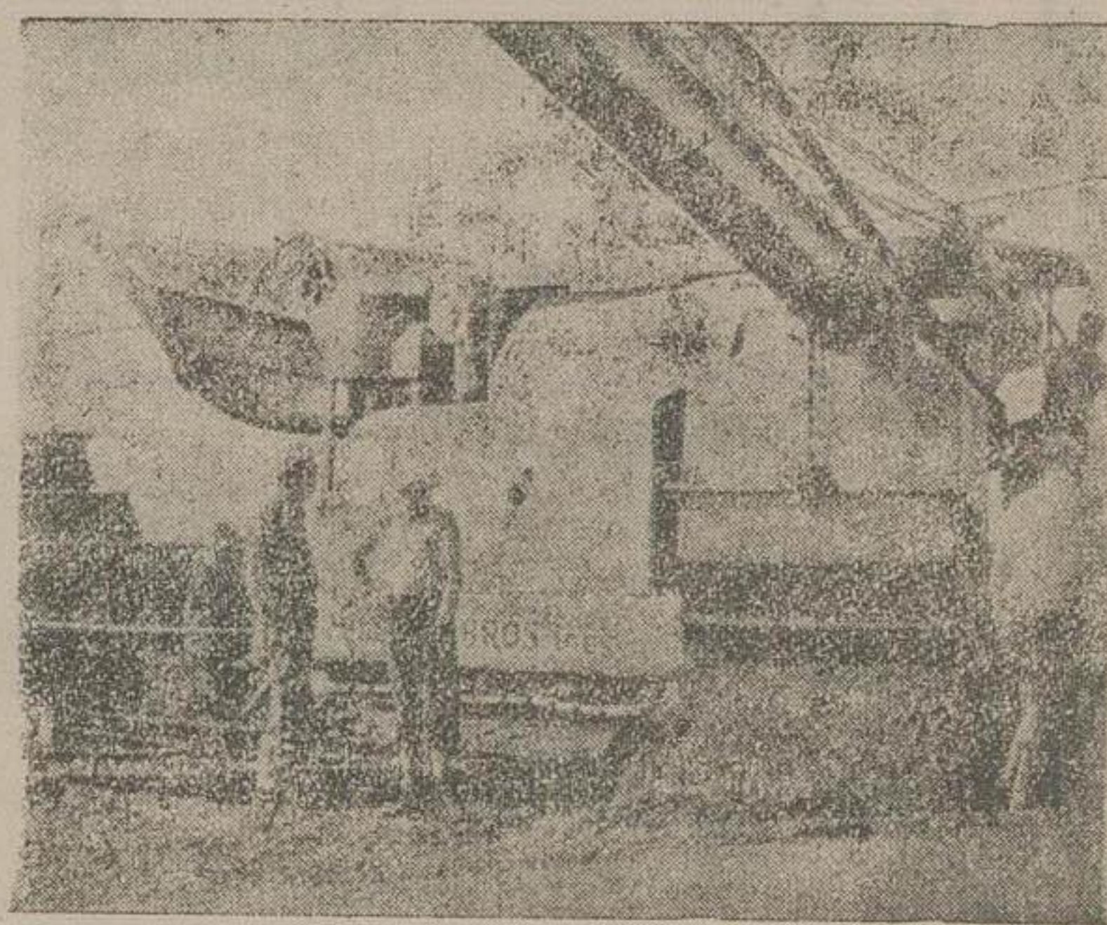
ماشین اسیاب و ریوی رگس REX PAVER
