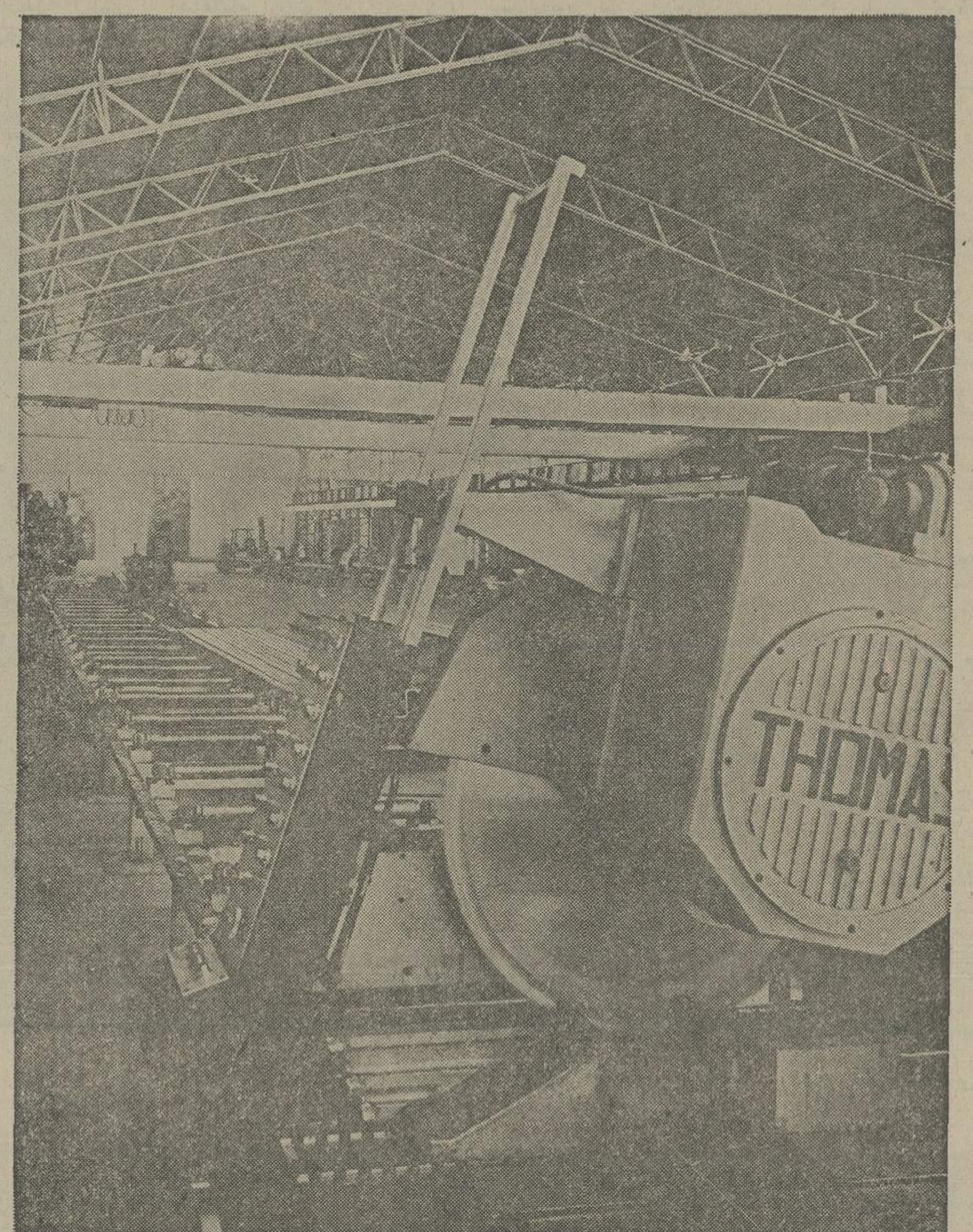
قسمت برش اتوماتیک کارخانه فولادی پارس
