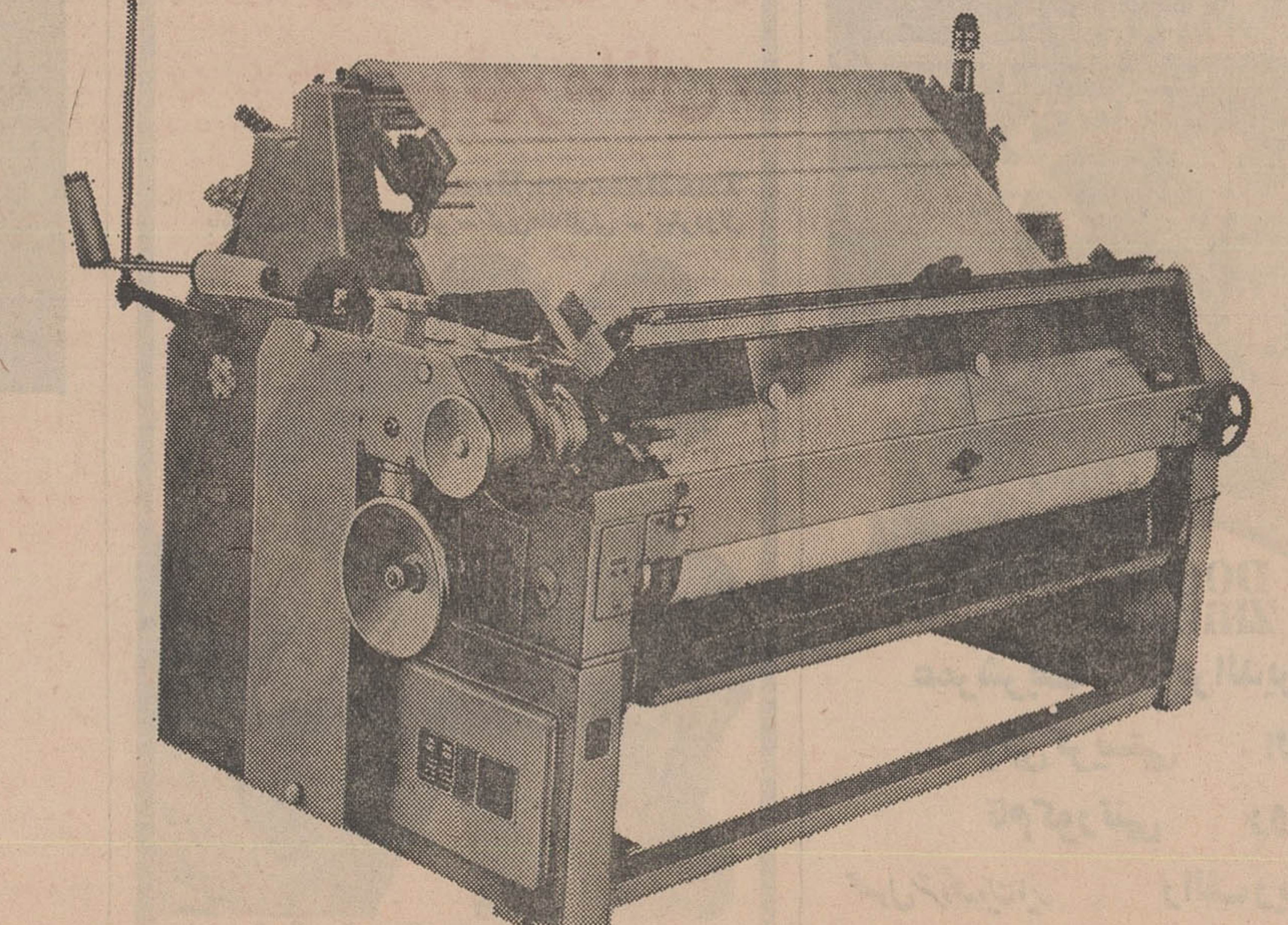
ماشین بافندگی جت هیدرولیک
