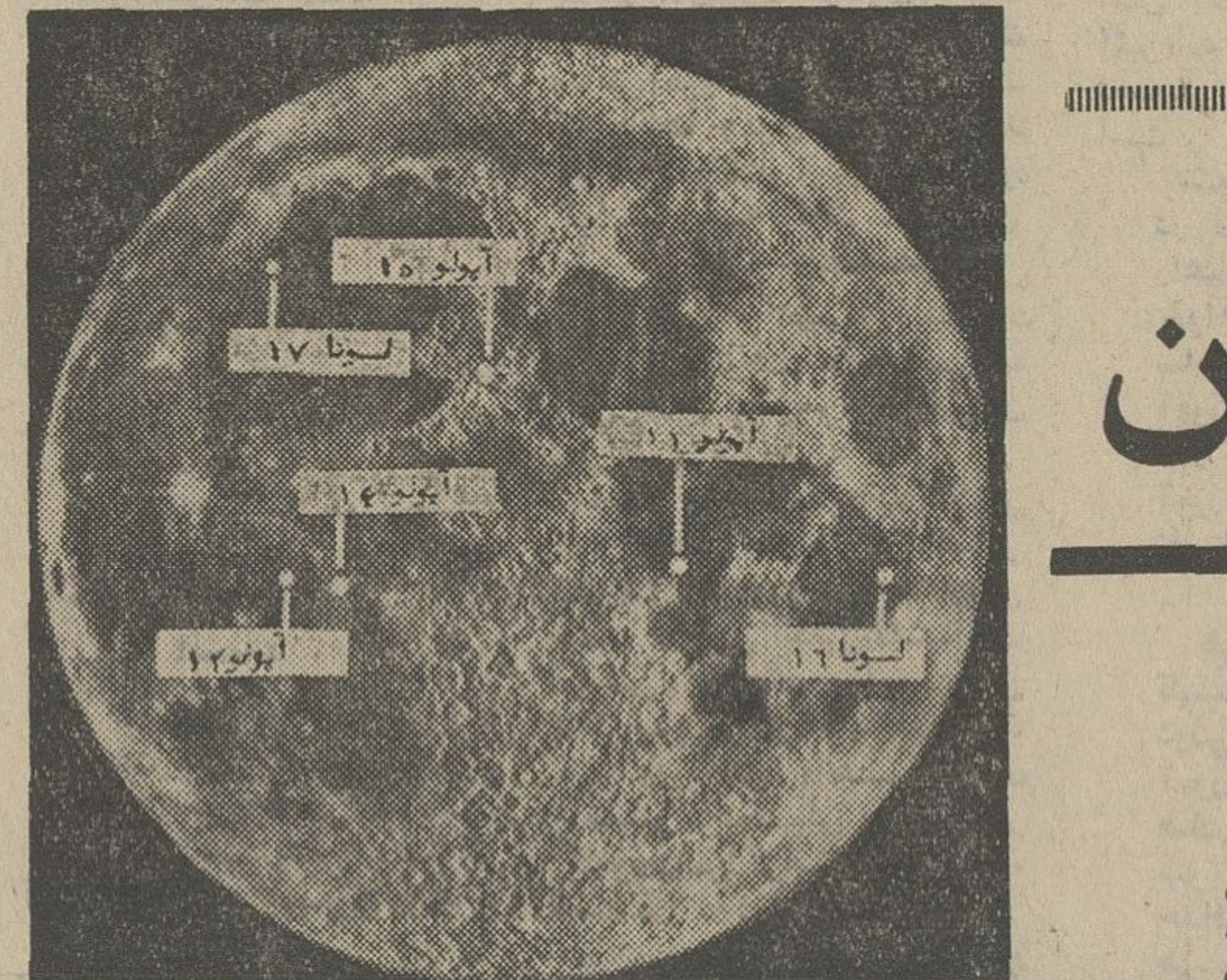
در عکس نقطه ای از کره ماه که سفینه ماه نشین آپولو ۱۵ در آن فرود می آید مشخص شده است نقاطی که سفاین روسی و امریکایی قبلا در آن فرود آمده اند نیز در عکس دیده میشوند .
