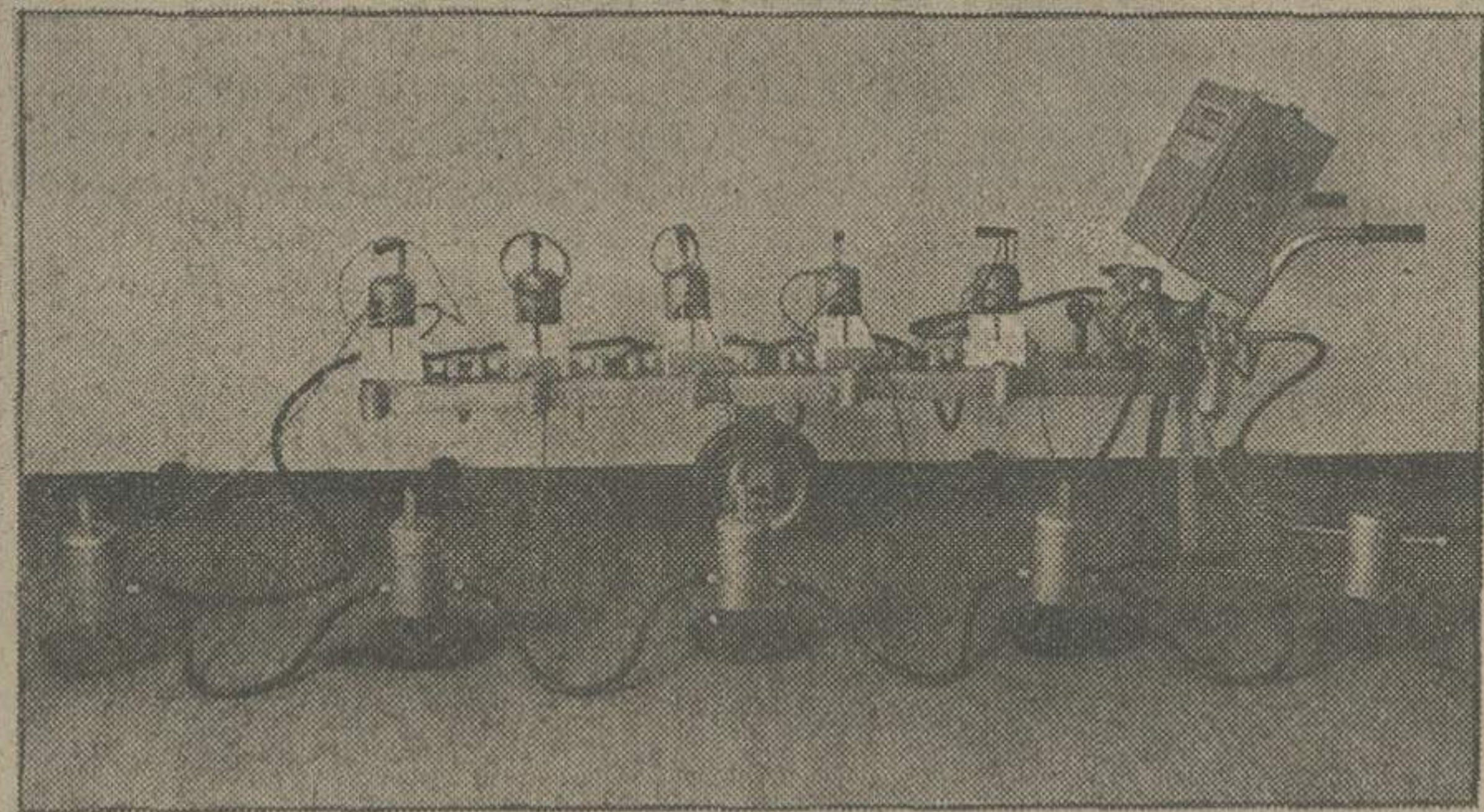
سوخت پاش «ایپالس» ترمو
