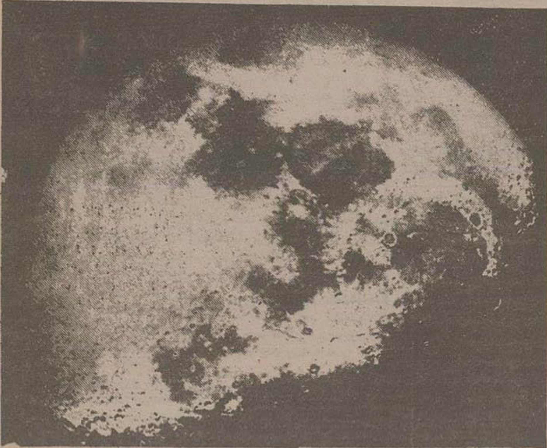
این عکس بوسیله تلسکوپ عظیم کپ کانورال مرکز موشکی آمریکا برداشته شده است و نیمه‌ای از ماه را نشان می‌دهد که از زمین دیده میشود. قرار بود که قمر مصنوعی آمریکا اطلاعاتی از نیمه نامرئی ماه زمین بخارند کند
