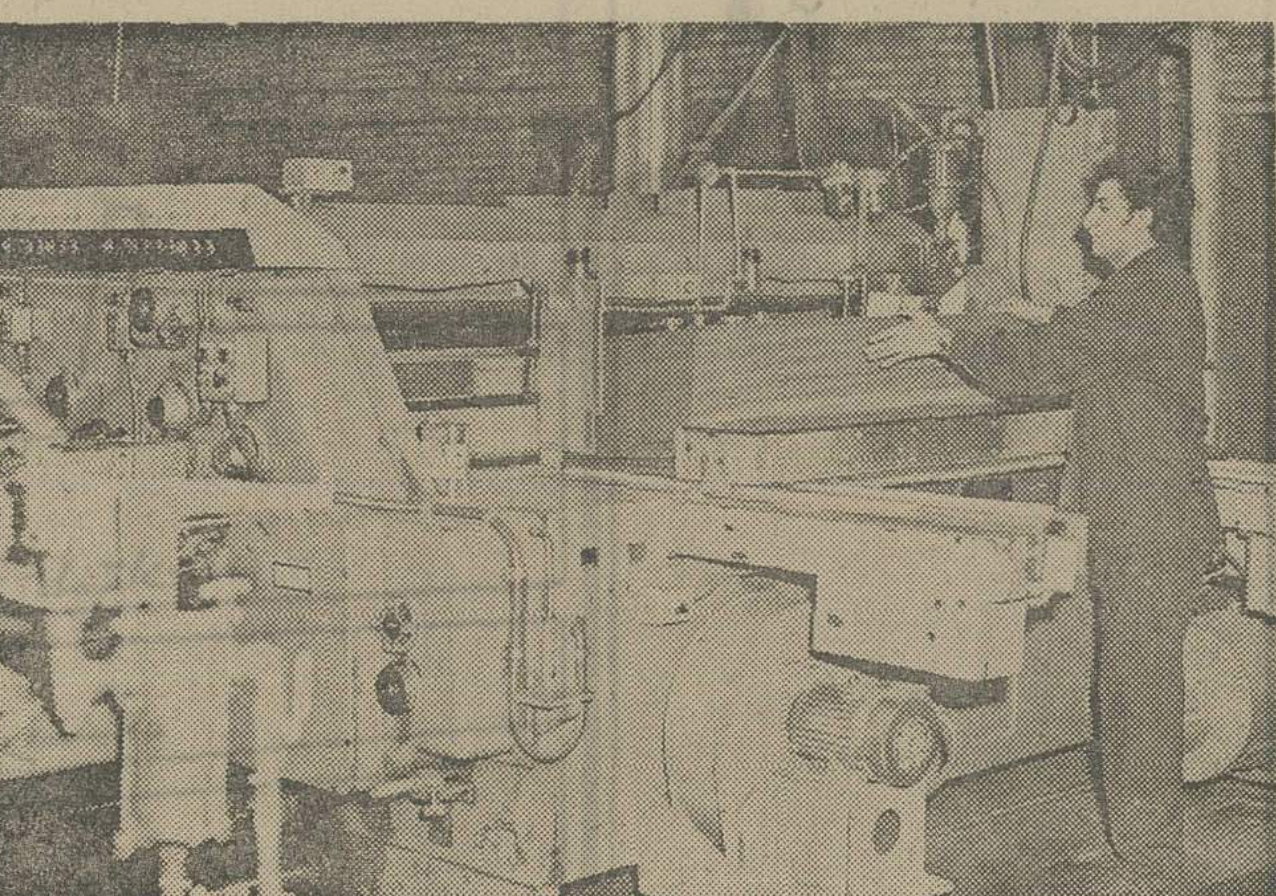
ماشین چاپ فلکسور که با دستگاه های چسب و بسته بندی مجهز بوده و قادر است، ورق‌را بصورت اتوماتیک تبدیل بکارتن نماید.
