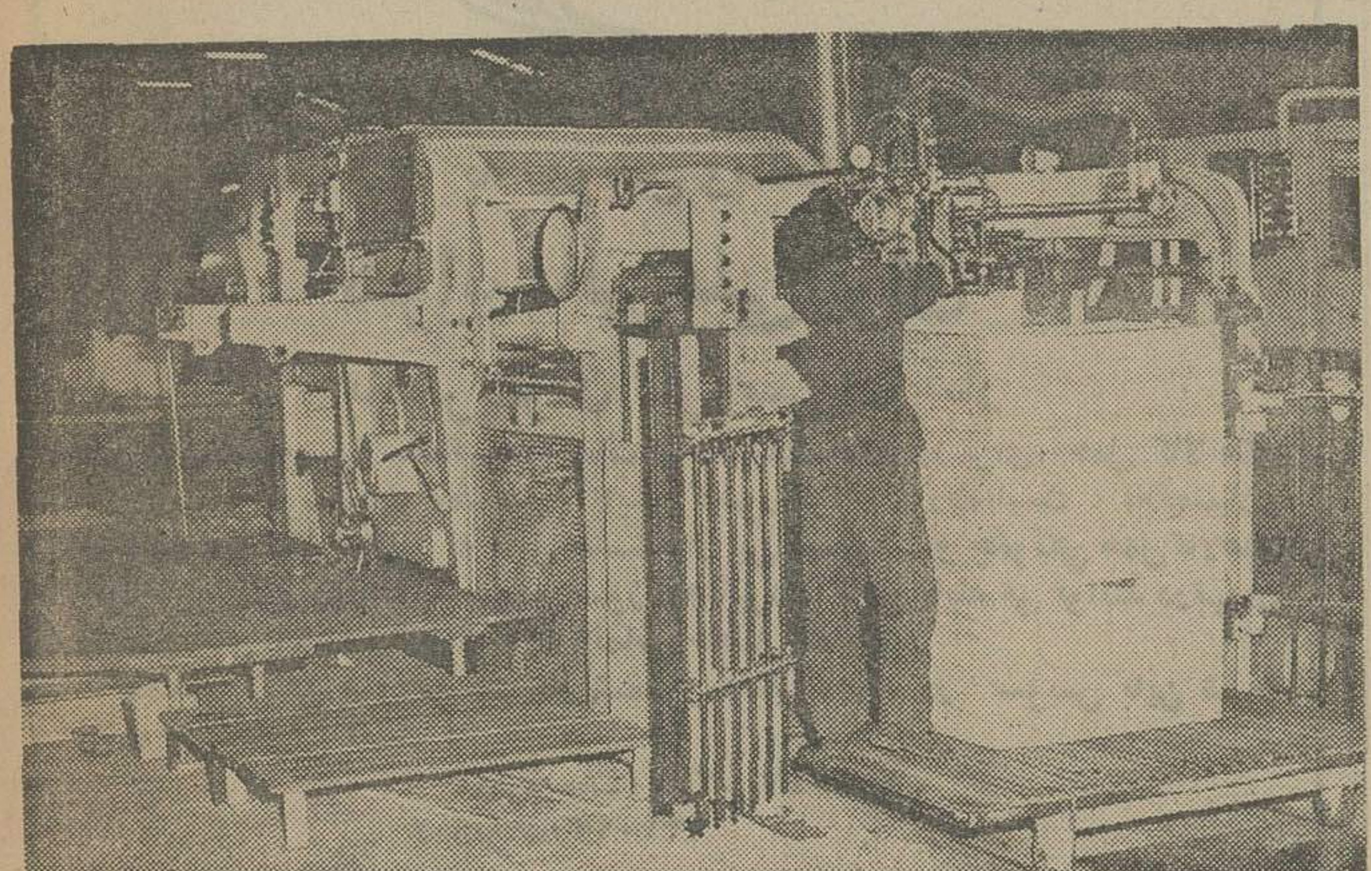
ماشین وایکات مدل SPE که از ورق باشکل های مختلف جعبه میسازد.
