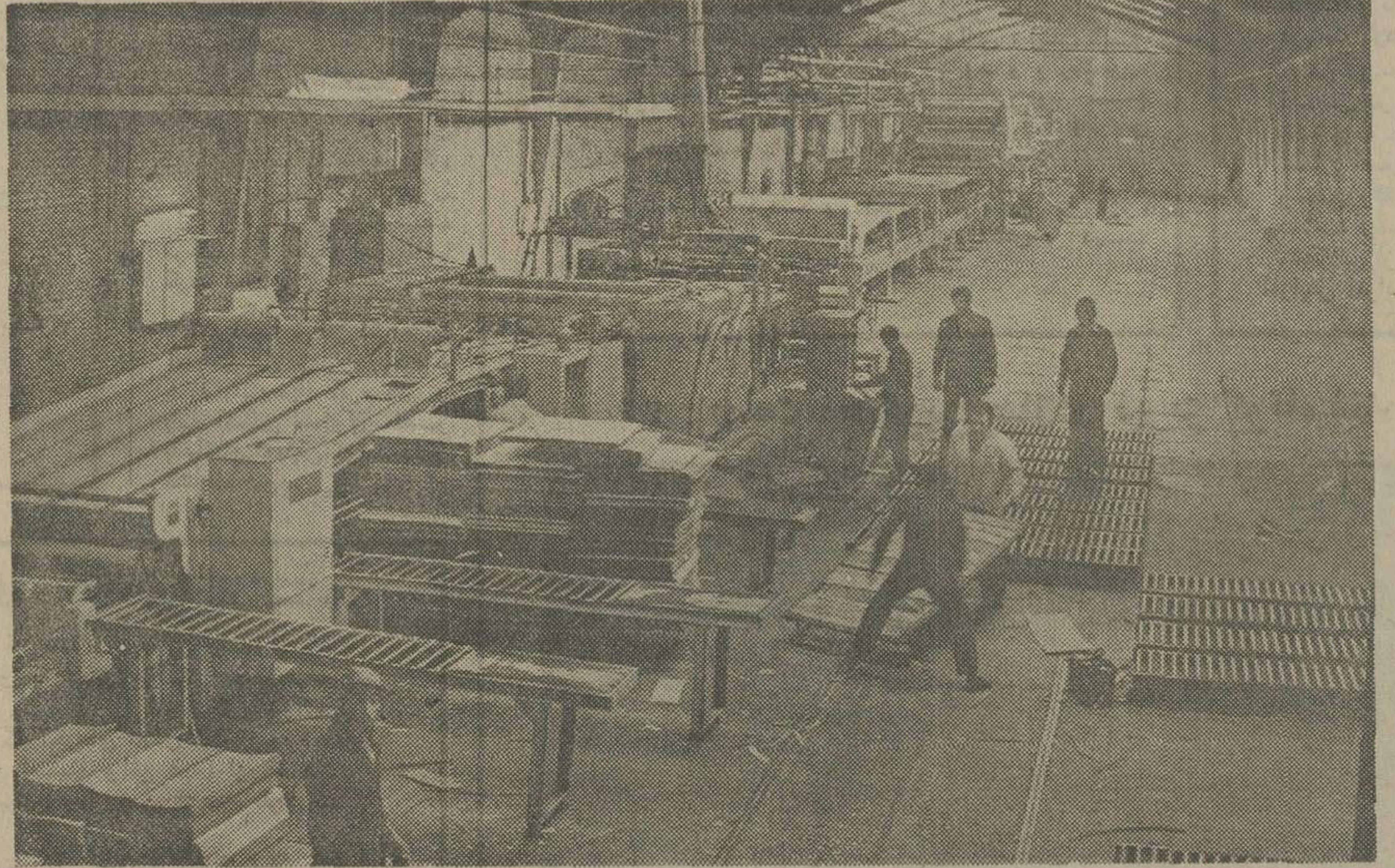
ماشین مقواسازی لنگستون مجهز به دستگاه های سازنده کنگره C و B مخصوص ساخت کارتن برای صنایع سنگین.
