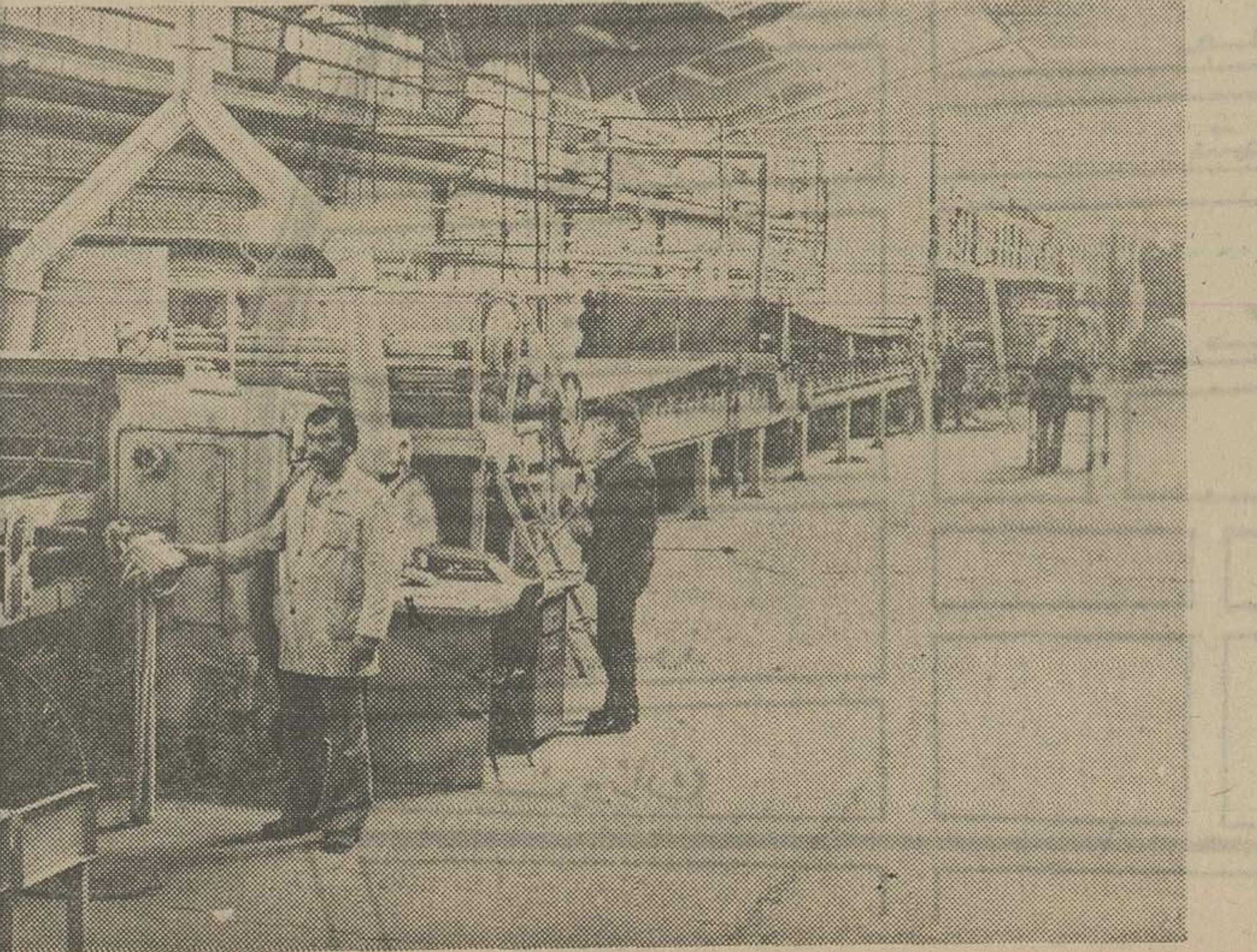
ماشین غول پیگرمقواسازی پیترز مجهز به ماشین های سازندکنگره B.E مخصوص ساخت متوا های طریف.
