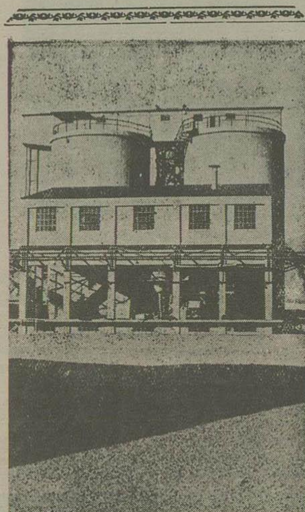
سیلوهای ذخیره سیمان و دستگاه بسته‌بندی سیمان در پاکت‌های پنج لا حاضر و آماده کار است
