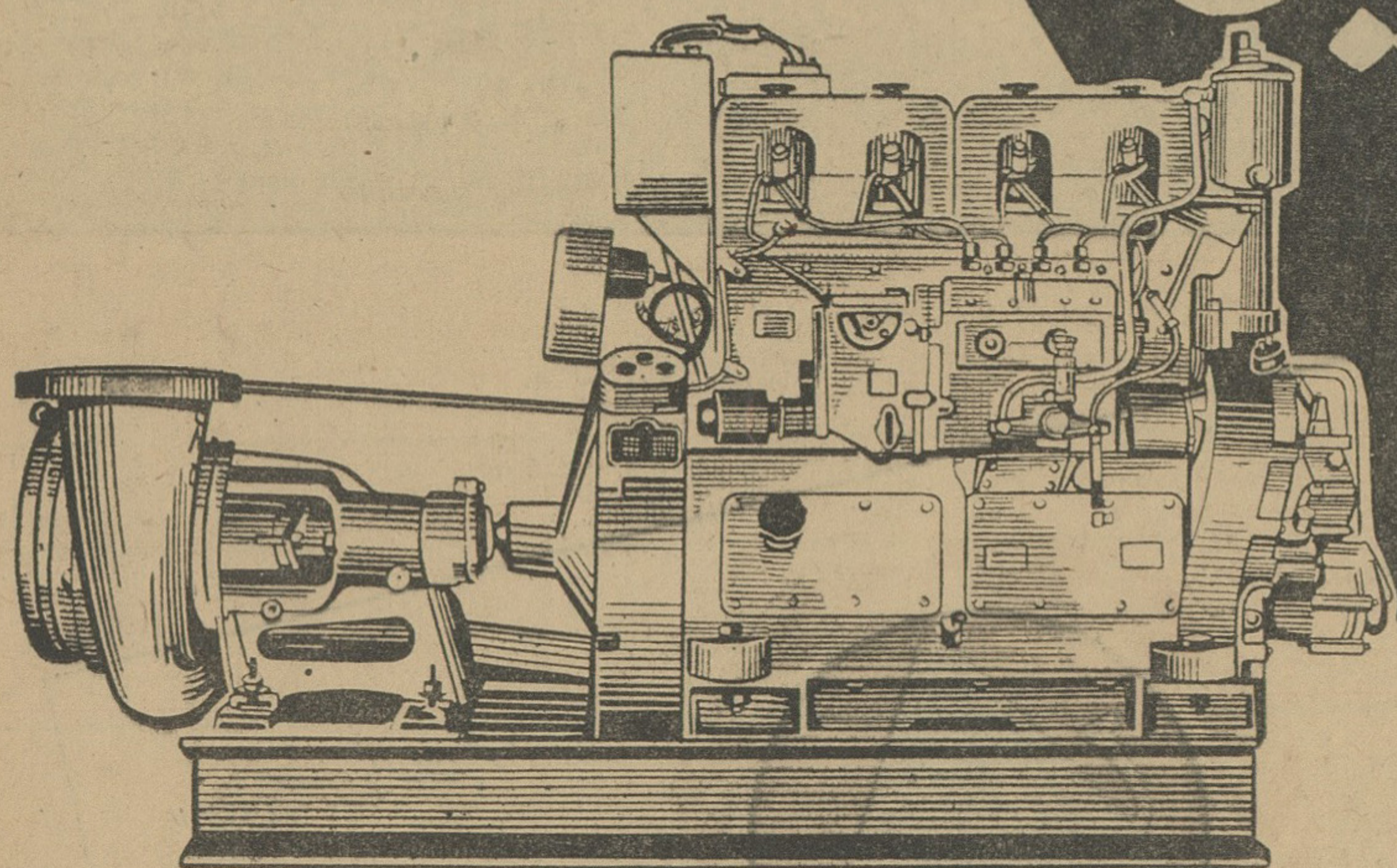
موتور پمپ دیزلی بقدرتهای مختلف از ۳ تا ۱۴ اسب
