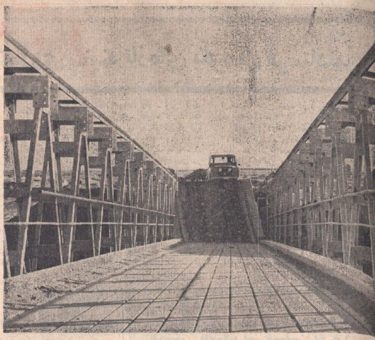
نمایی از پل شکسته محمدآباد که بوسیله خبرنگاران تهیه شده و در آن وضع پل پس از نشست نشان داده شده است
