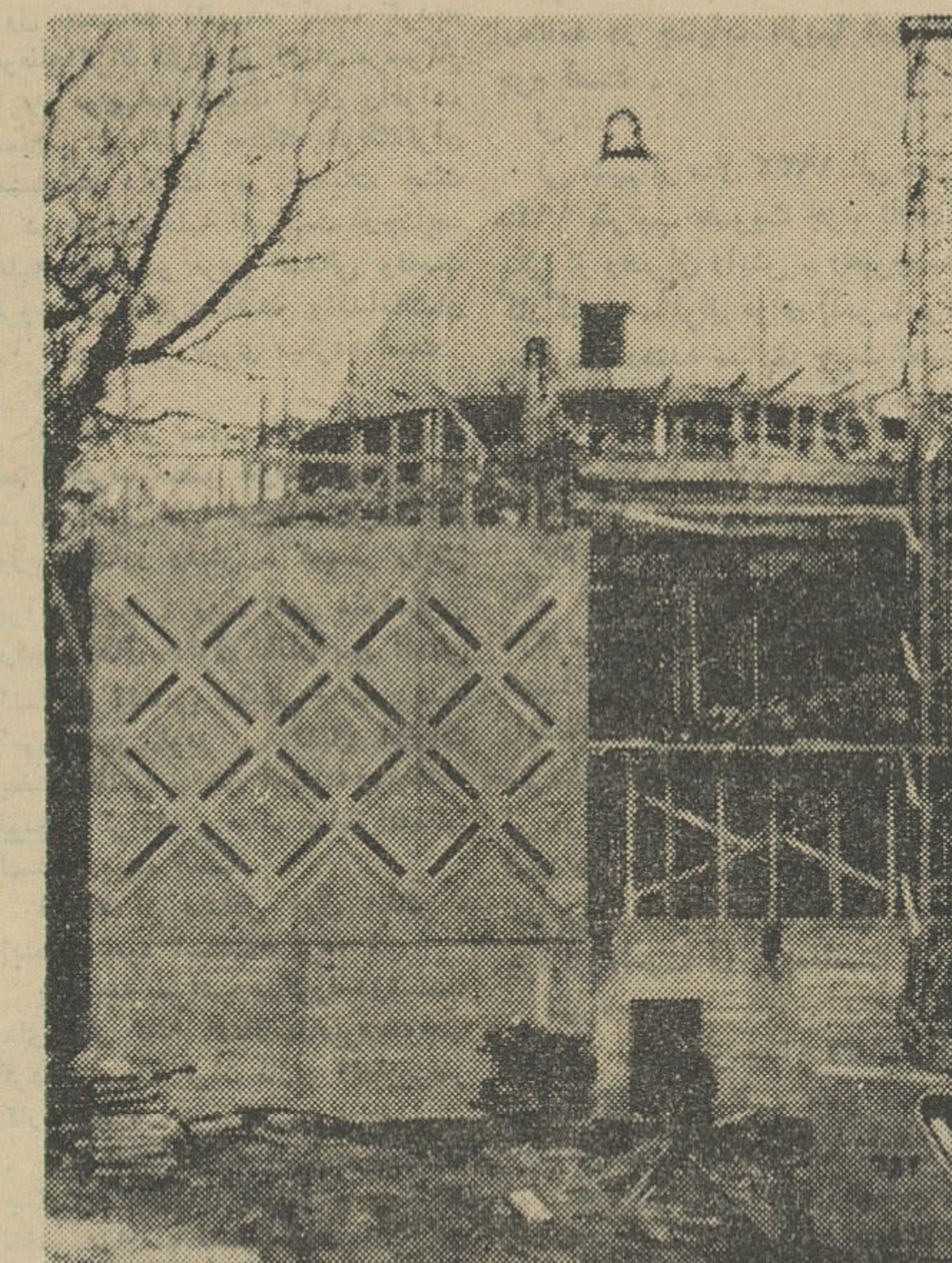
زیر سازی و اسکلت بنای مسجد ایرانیان در هامبورگ
