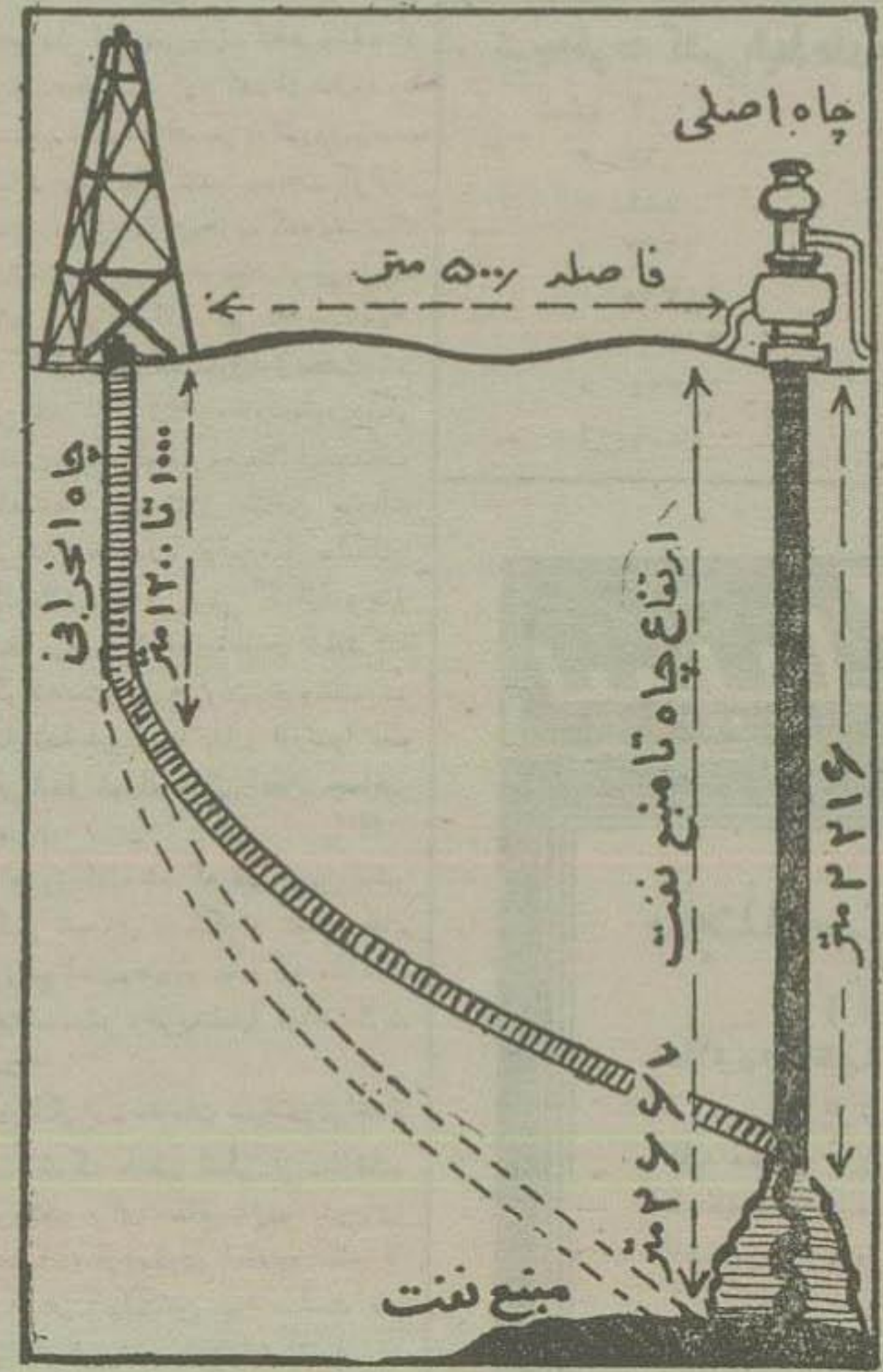
نقشه چاه انحرافی که در کنار چاه شماره ۵ حفر میشود
