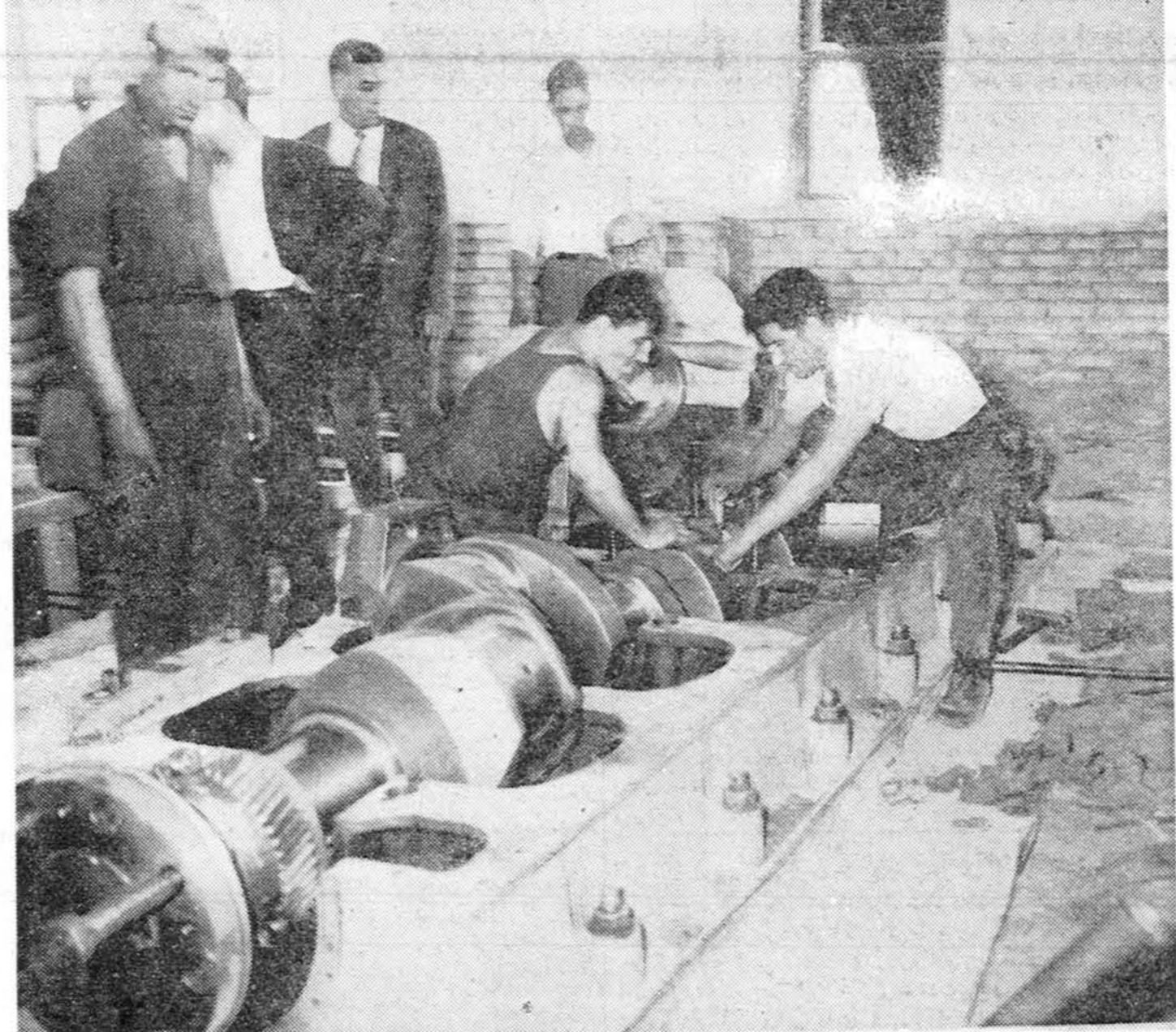
اینجا ساختمان کارخانه جدید برق شهاب است این کارخانه در شمال پادگان جی ساخته شده و مامورین بطوریکه ملاحظه میشود مشغول نصب موتور میباشند این موتور دارای پانصدکیلووات نیرو است و فعلا دو دستگاه از آن در کارخانه جدید نصب میشود
