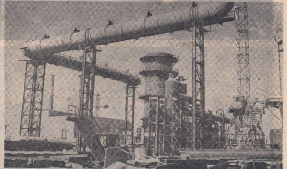
کوره بلند، تصفیه گاز
