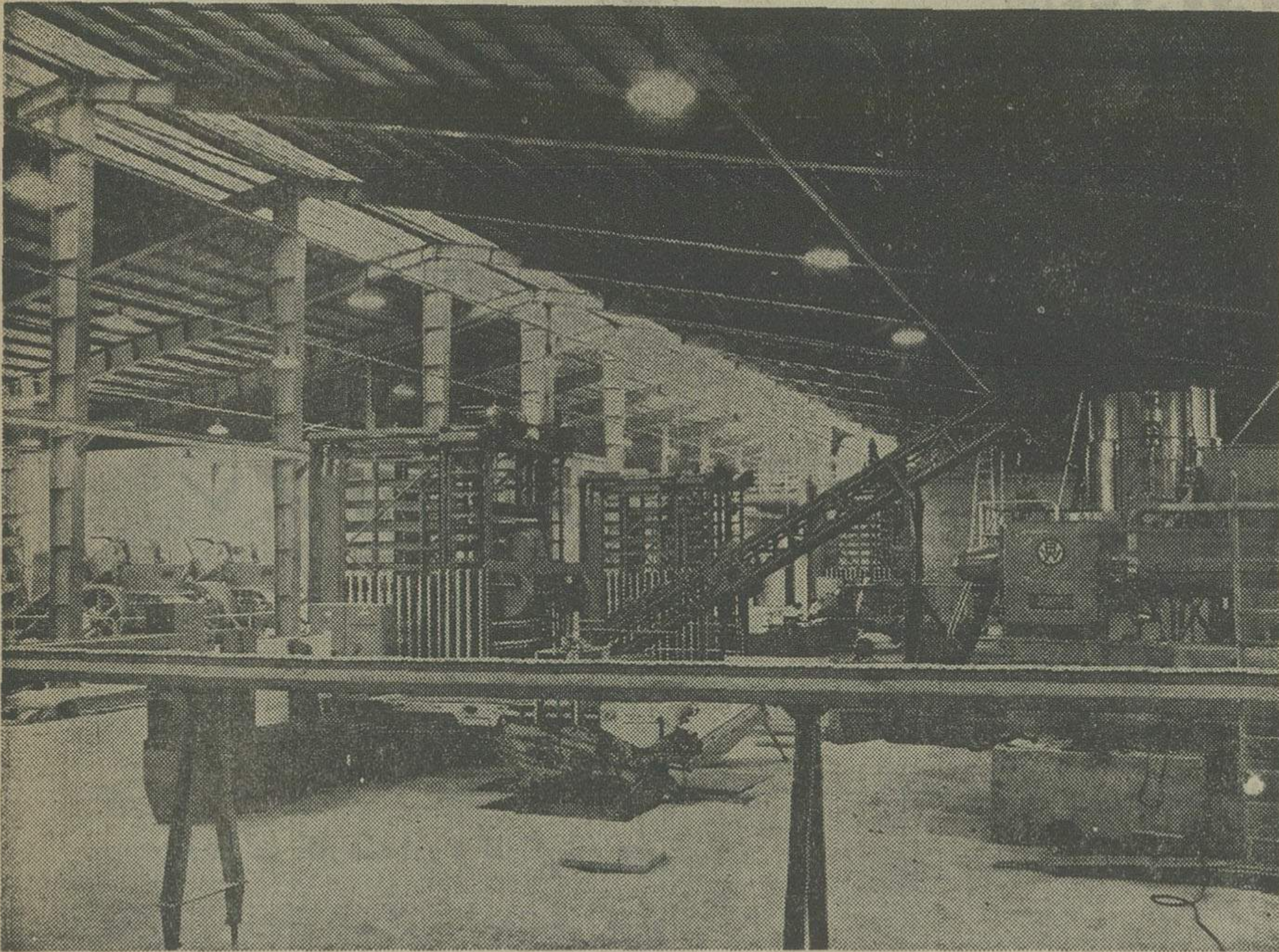
این قسمتی از ماشینهای آماده کردن گل در کارخانه است این ماشین تمام اتوماتیک و ساخت کارخانه «ریترورک» RIETTERWERKE آلمان است
