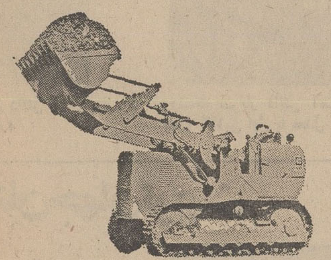
لودرهای چرخ زنجیری بقدت های ۷۰ الی ۲۷۵ قوه اسب ظرفیت ذبه از یک الی ۳/۵ متر مکعب
