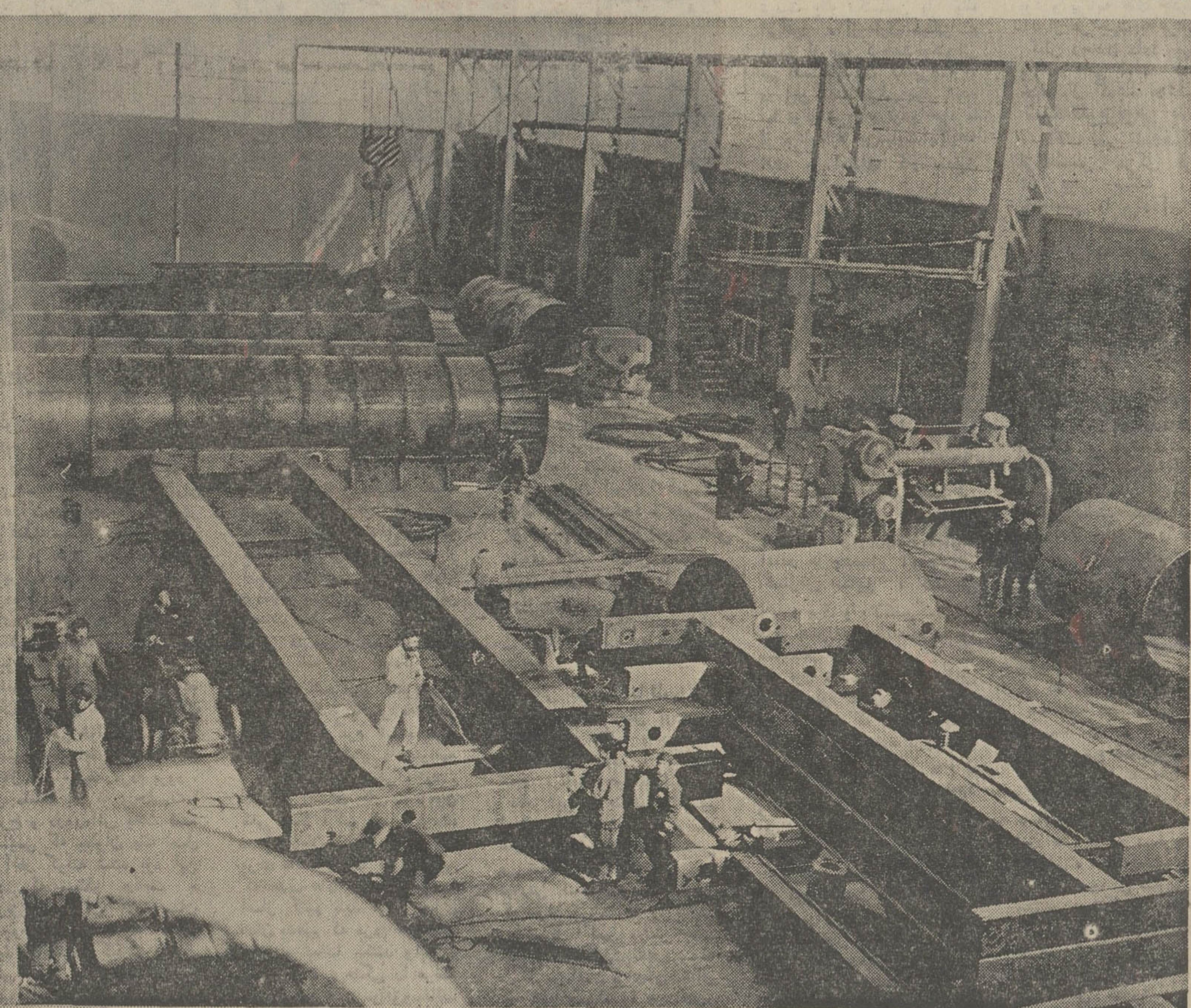
یکی از سالن‌های کارخانه «فیروز» که عملیات مربوط به شادولوله گاز در آن ساخته و پرداخته میشود
