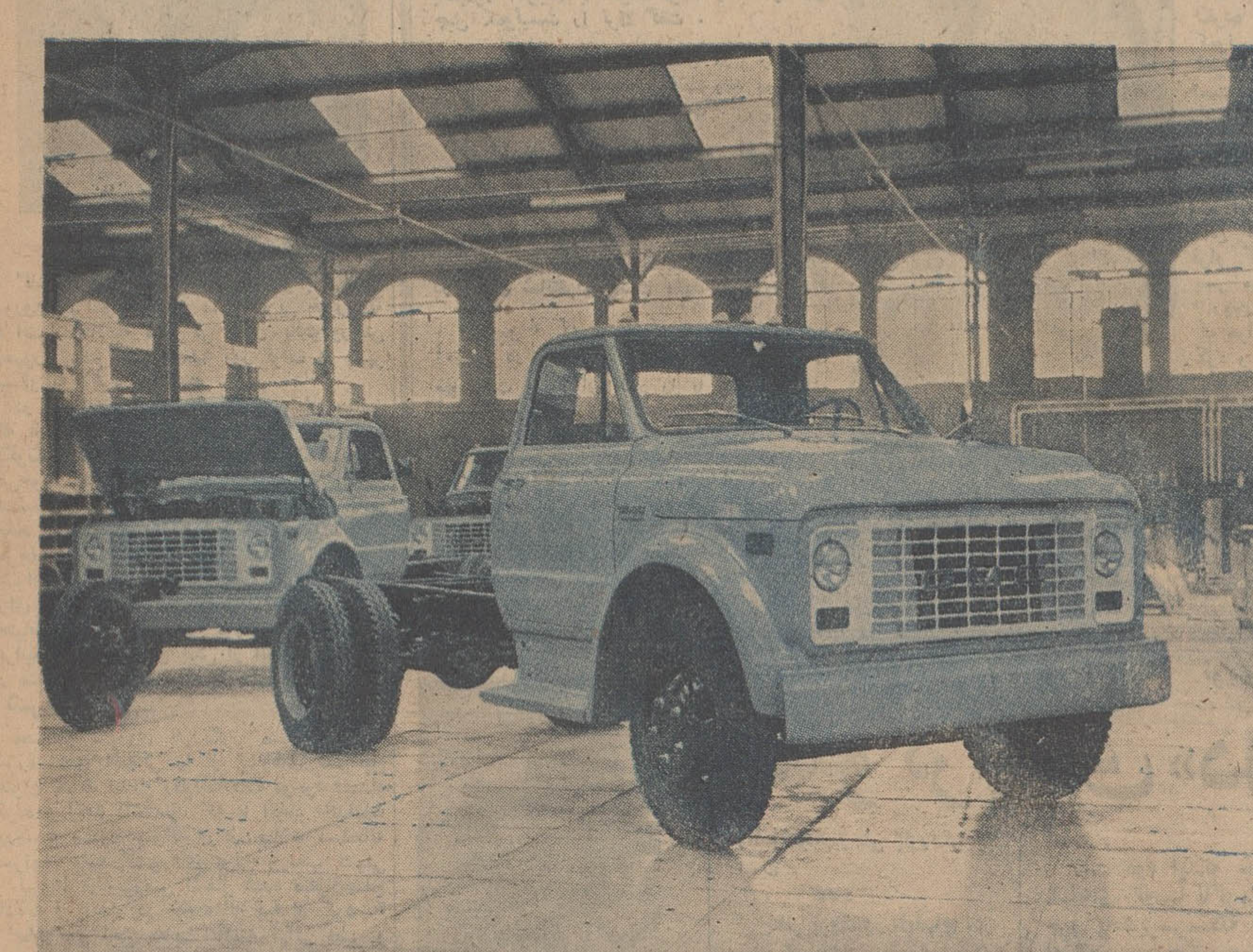
طاق این کامیونت جهس در کارخانجات شرکت ایران کاوه از ماده جدید ورقبب سرسخت فولاد «فایبرگلاس» ساخته شده است.
