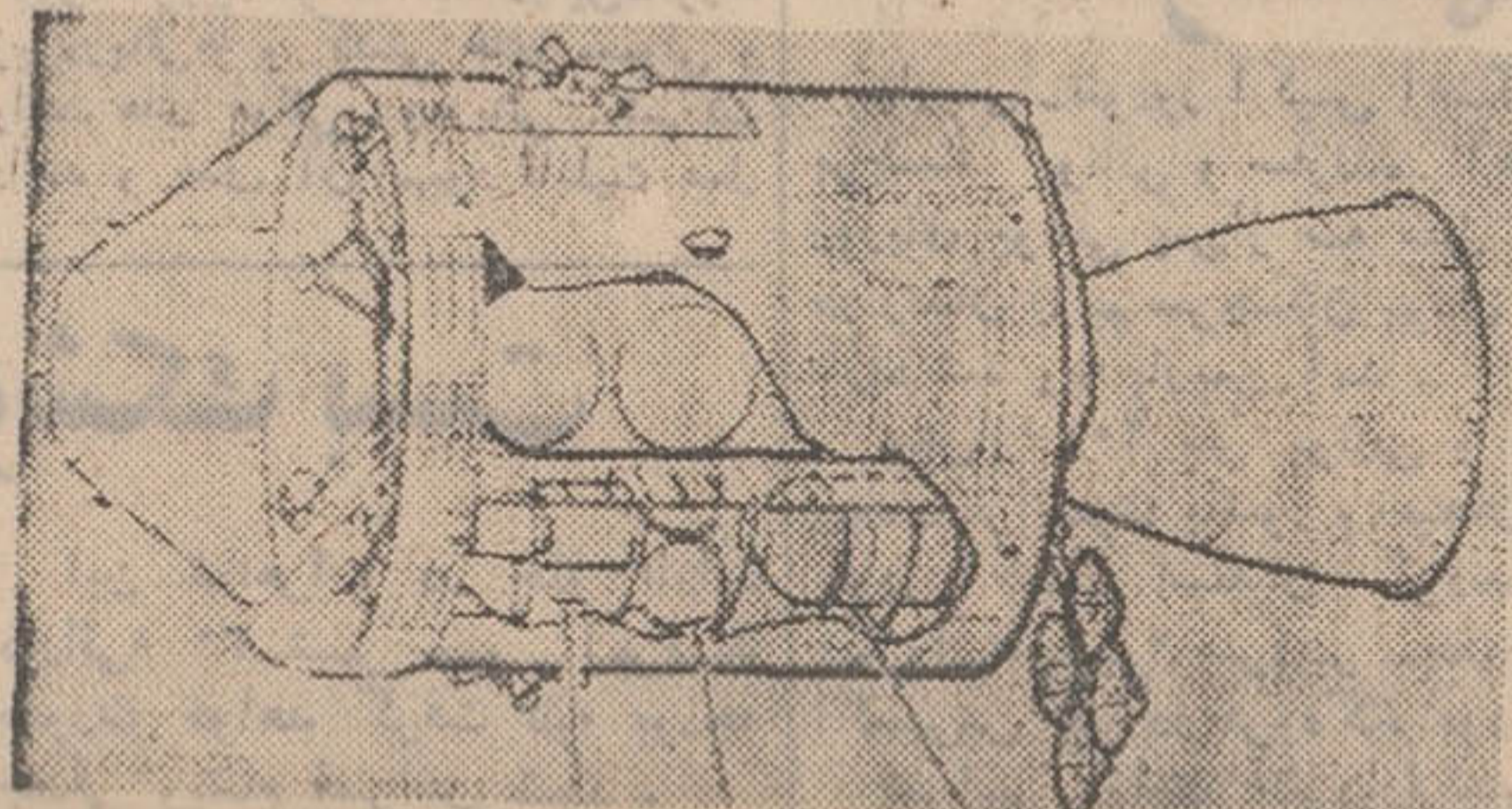
در این تصویر نقشه سیستم فرماندهی آپولو ۱۳ و سفینه ماه نشین و مخازن سوخت آن که سوراخ شده نشان داده شده است. عکس رادیویی اطلاعات
