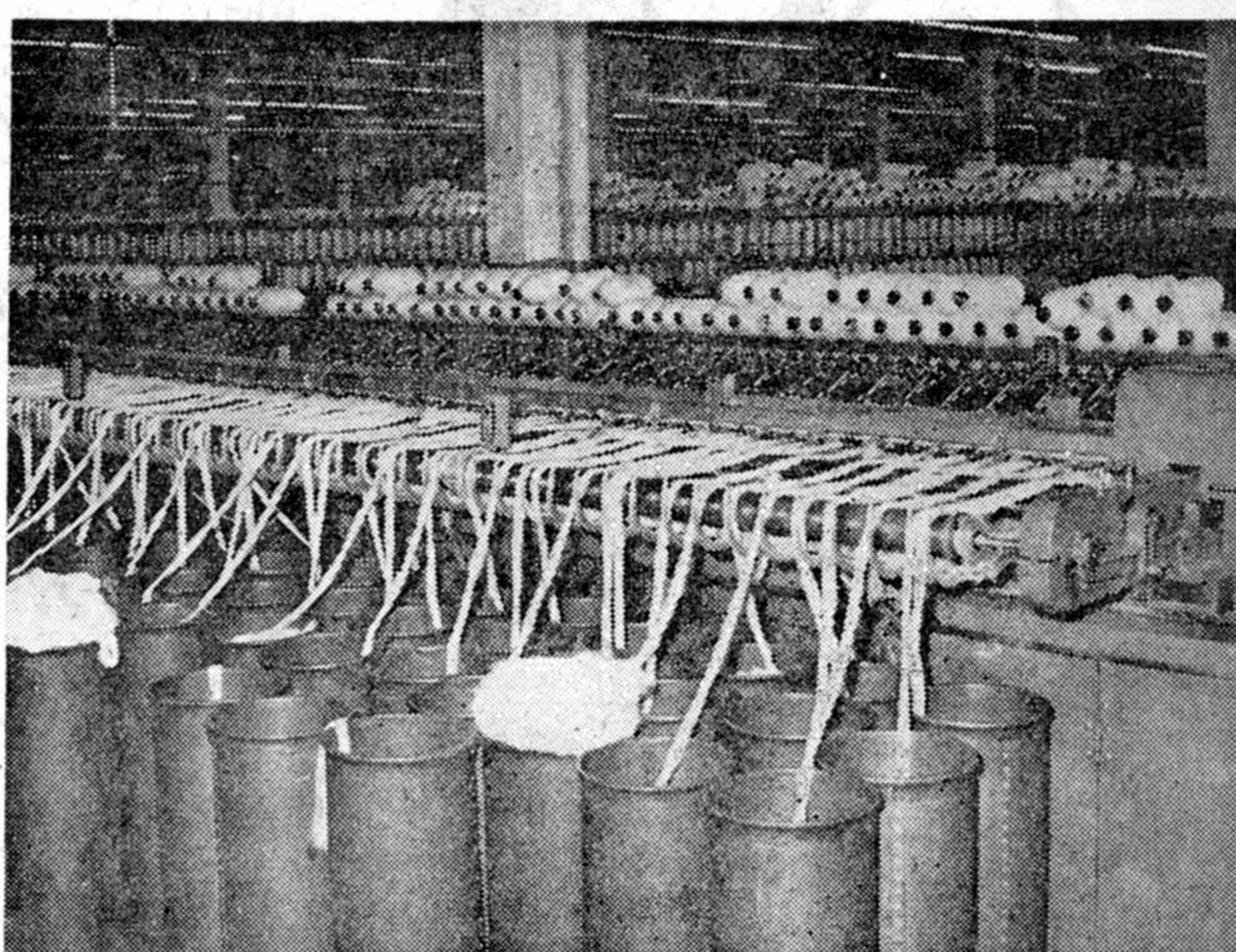
نمای قسمتی از سالن ریسندگی نیم تاب ماشینهای و ماشینهای اتوماتیک آن
