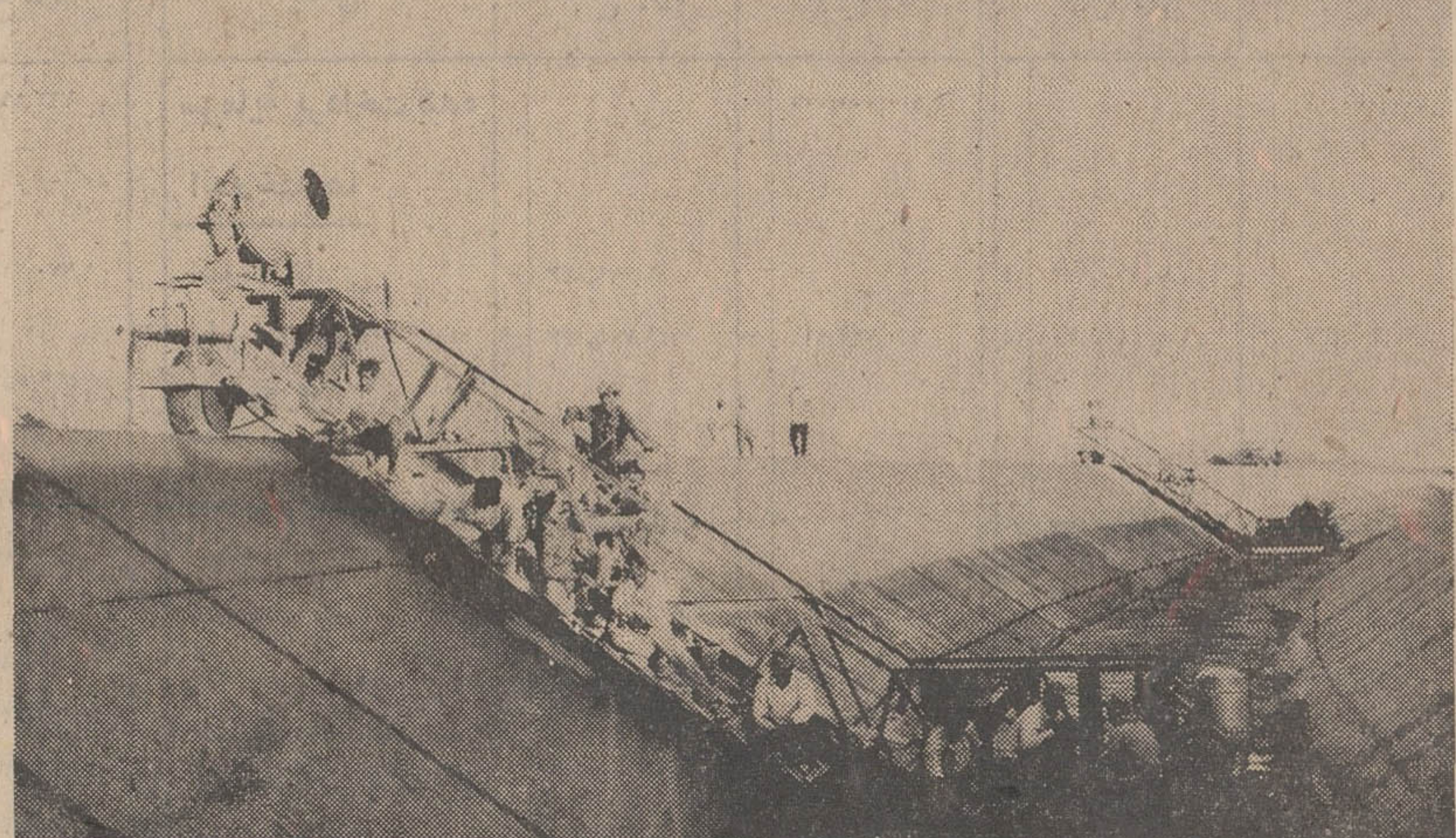
این ماشین غول بیکر بطور اتوماتیک کانالهای آبیاری طرح دز بزرگ را بتون ریزی میکند.
