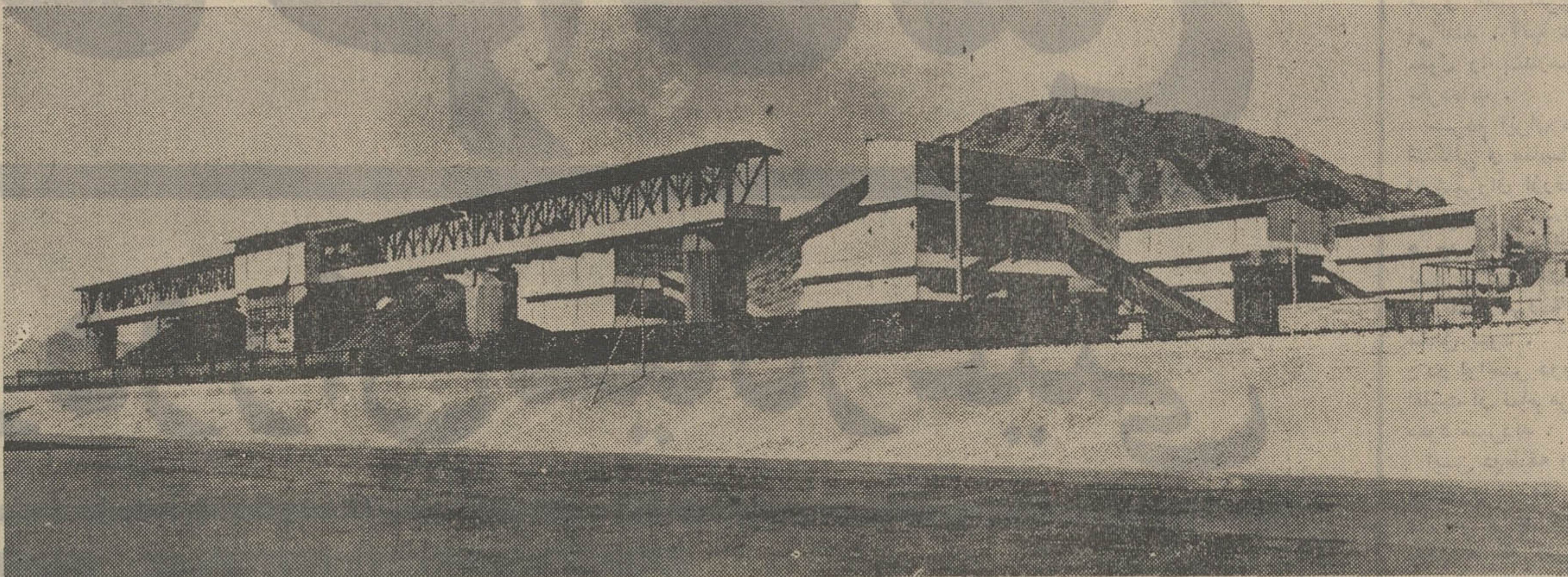
نوار بارگیری که بعد از آخرین سنگ شکن قرار گرفته است. سنگ آهن پس از چرخیدن در محله خرد شدن در سنگ شکنهای مختلف زیر نوار بارگیری باران بند می آید که با نوار بارگیری دیگر به کارخانه حمل می گردد.
