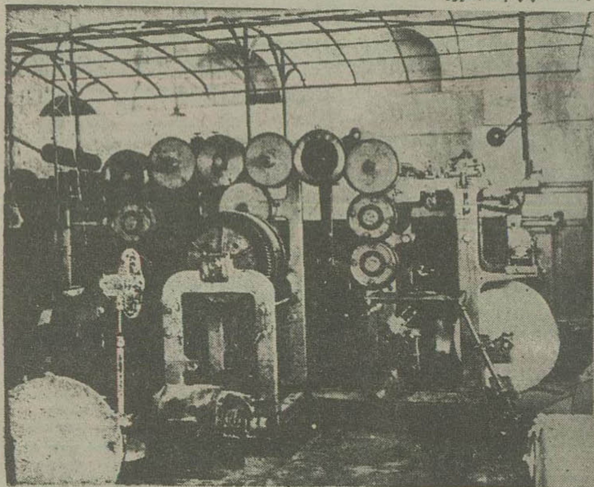
«رتاتیو» بزرگ اطلاعات که سیزده متر طول و دویست و نود ارتفاع آنست با نصب دستگاه تکمیلی جدید میتواند بیست و چهار صفحه روزنامه را با پنج رنگ مختلف حداقل سی هزار شماره در ساعت چاپ آماده کند - این ماشین آخرین اختراع در صنعت چاپ بشمار میرود
