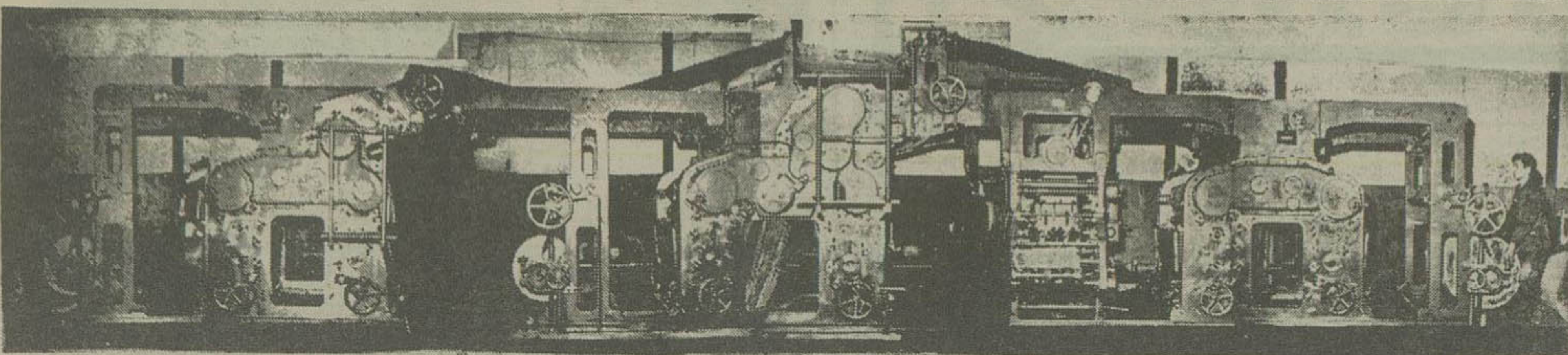
«رتاتیو» بزرگ اطلاعات که سیزده متر طول و دویست و نود ارتفاع آنست با نصب دستگاه تکمیلی جدید میتواند بیست و چهار صفحه روزنامه را با پنج رنگ مختلف حداقل سی هزار شماره در ساعت چاپ آماده کند - این ماشین آخرین اختراع در صنعت چاپ بشمار میرود
