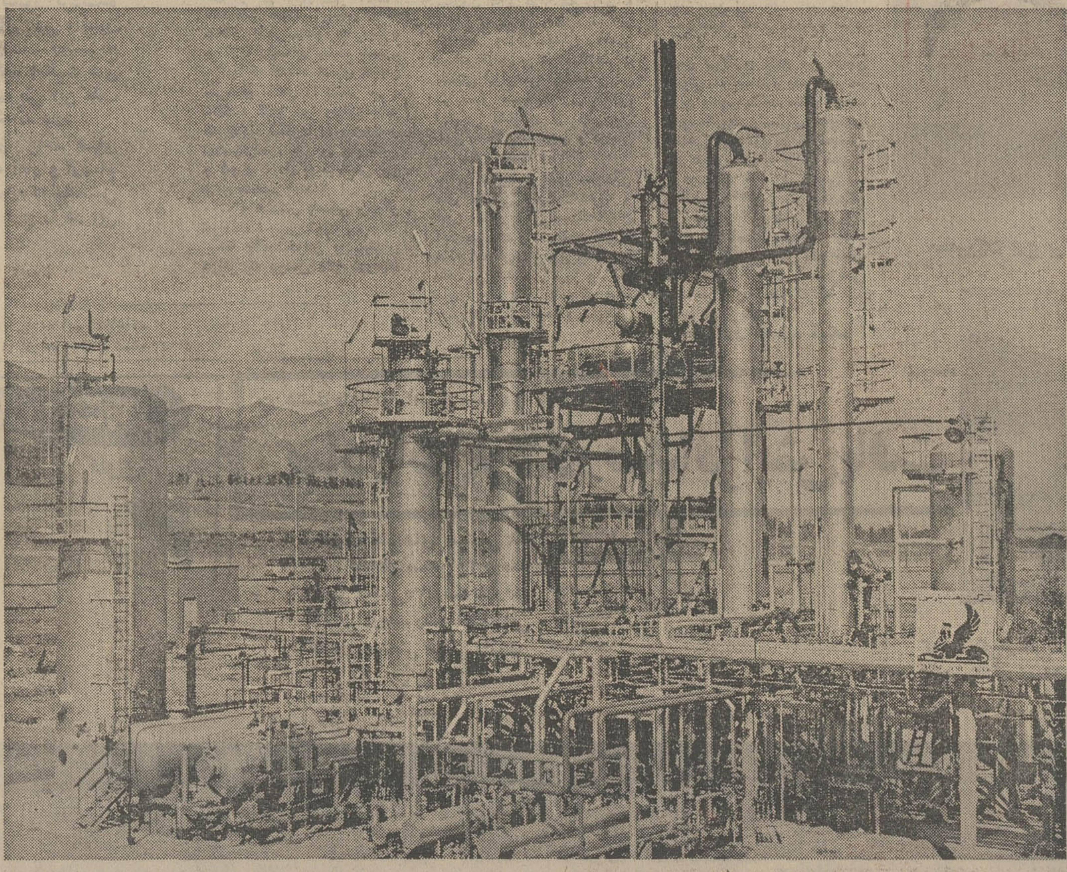
نمای قسمتی از دستگاه فورفورال (تصفیه - روغن) شرکت نفت پارس .
